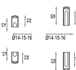
2314 set copricerniere corto piatto 16mm flat short cover hinges set 16mm
